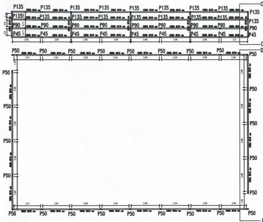
1 DETALHAMENTO DA ESTRUTURA DE CONCRETO - FECHAMENTO SUPERIOR ESCALA INDEFINIDA
