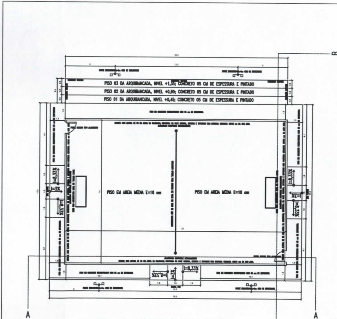
1 PLANTA BAIXA COMPLETA DA QUADRA DE AREIA ESCALA INDEFINIDA
