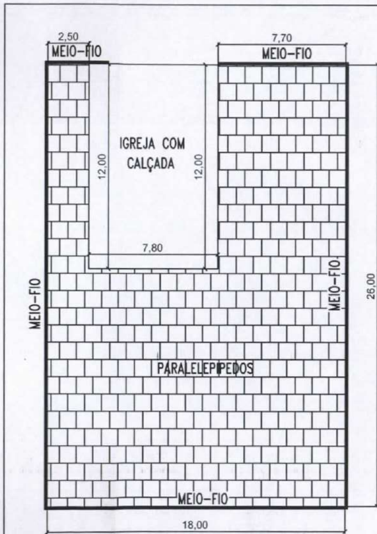
1 PLANTA BAIXA ESCALA (SEM ESCALA)
