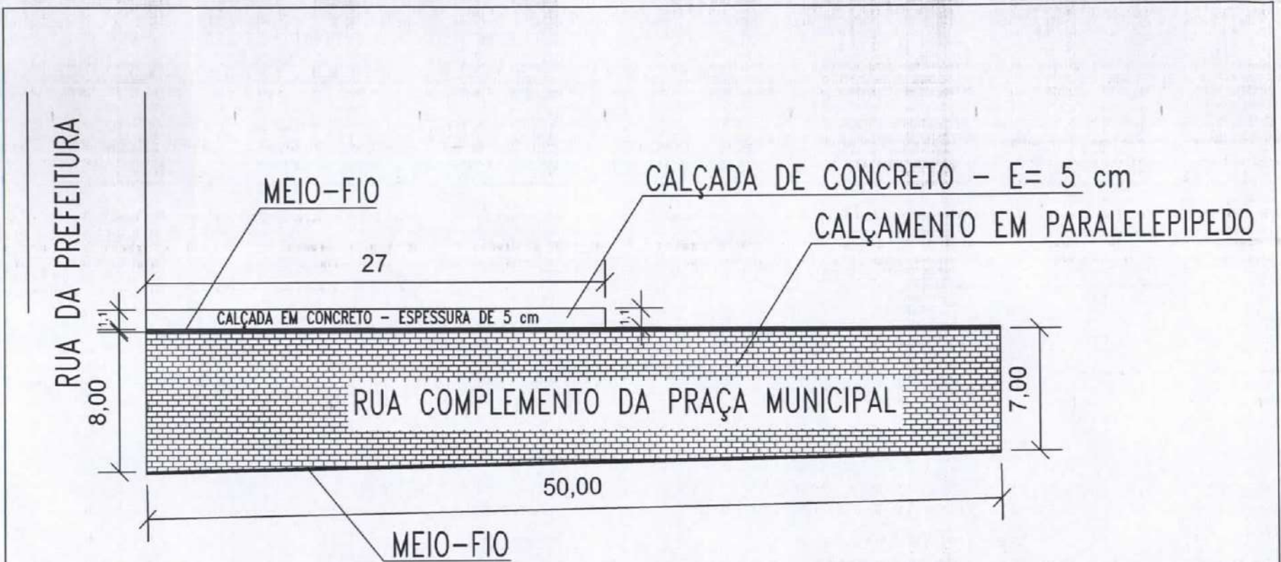
1 DETALHAMENTO DA RUA A SER PAVIMENTADA ESCALA INDEFINIDA
