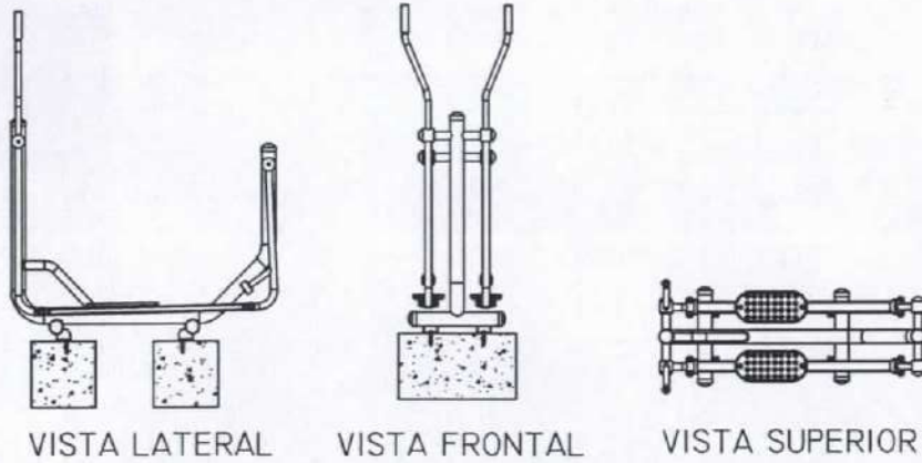
1 DETALHAMENTO DO ESQUI INDIVIDUAL ESCALA INDEFINIDA
