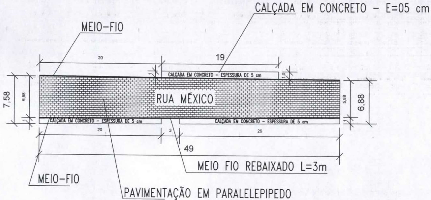
1 DETALHAMENTO DA RUA A SER PAVIMENTADA ESCALA INDEFINIDA
