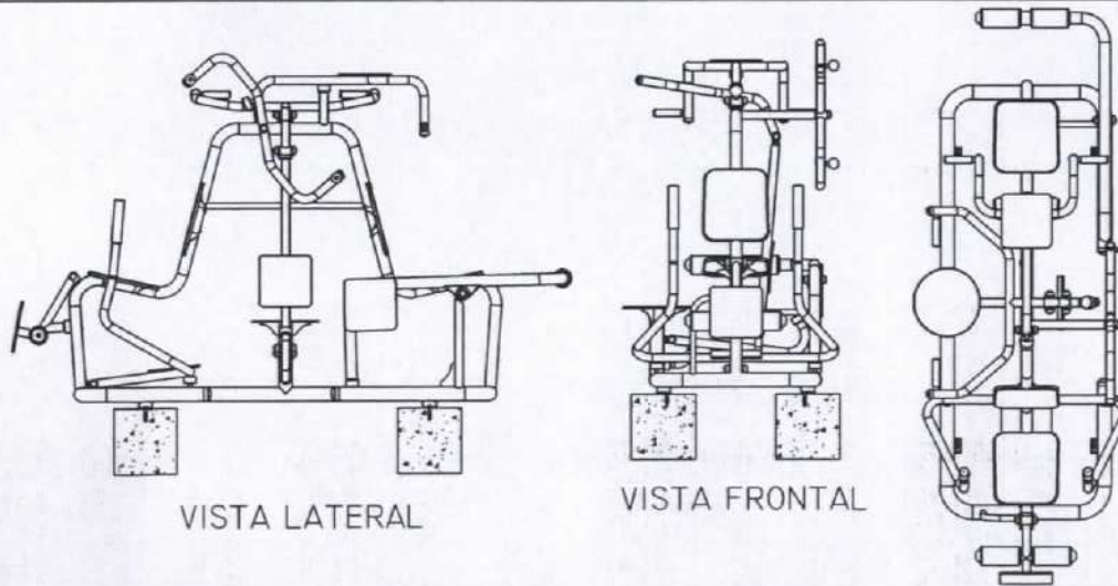
3 DETALHAMENTO DO MULTIEXERCITADOR 06 FUNÇÕES ESCALA INDEFINIDA
